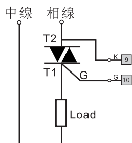
單相雙向SCR過零控制
