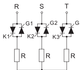
三相全控模塊
