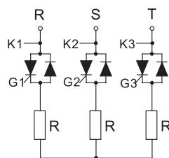
三相半控模塊
