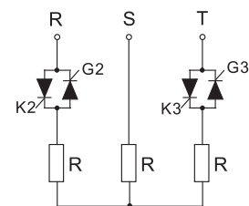
兩相全控模塊
