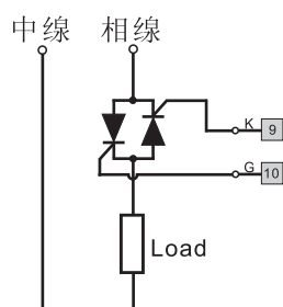
單相反并聯SCR過零控制
