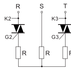
三相雙向SCR
